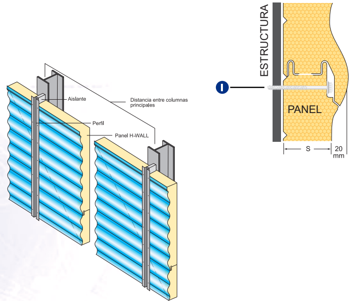
Detalle de la junta Longitudinal
